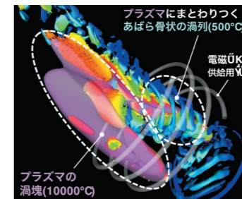
プラズマの渦塊(10000°C) プラズマ渦構造の理論的可視化の例(東北大学のスーパーコンピュータによって世界で初めて実現)
