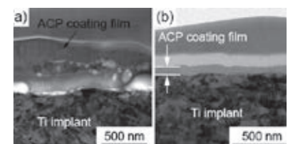
RFマグネトロンスパッタリング法により作製した非晶質リン酸カルシウム(ACP)薄膜 (a) および家兎大腿骨埋入1週間後 (b) の断面 Cross section of amorphous calcium phosphate (ACP) coating film fabricated by RF magnetron sputtering (a) before and (b) after 1 week implantation.
