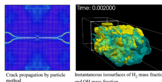
高圧水素タンク漏洩に発生したき裂伝播はばね物と着火を伴う反応性漏えい水素の拡散挙動に関する混相流-構造連成型コンピューティング Fluid-Structure coupled computing of crack propagation behavior in a high-pressure hydrogen tank bulkhead and diffusion behavior of reactive leaking hydrogen with ignition
