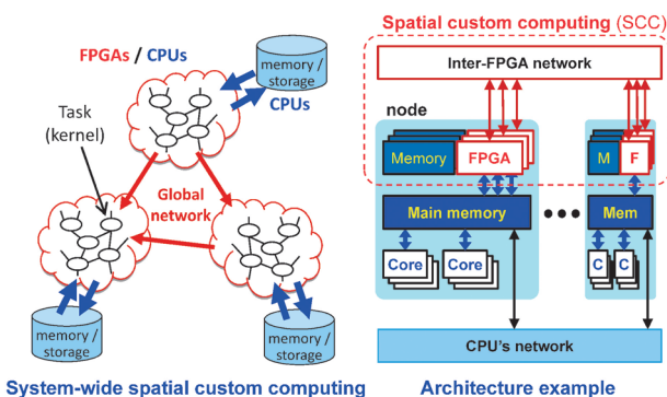
System-wide spatial custom computing Architecture example システム規模の空間的専用計算方式とその機構を有する先進的計算システムアーキテクチャの例
