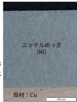
常温での ニッケルめっき組織
